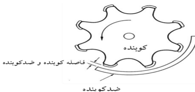
شکل ۴۷. فاصله کوپنده و ضد کوپنده. کم کردن بیش از حد این فاصله با این فرض که دانه‌های کنجد کوچک هستند موجب له شدن دانه‌های کنجد می‌شود. شکل از نویسندگان.
