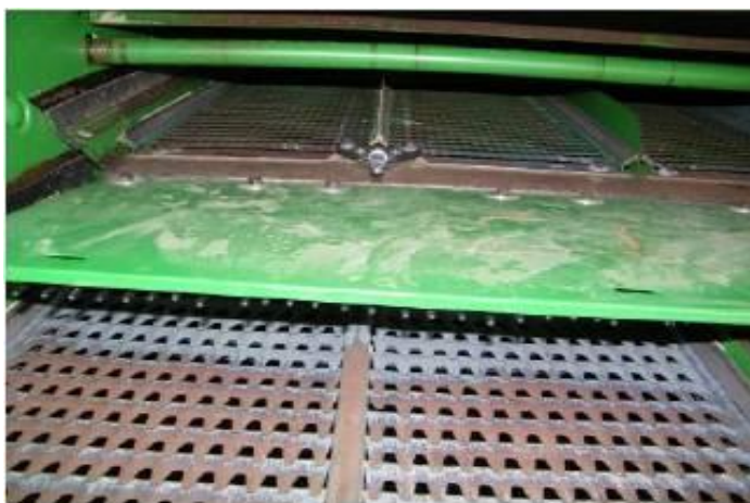
شکل ۴۸. مسدود کردن قسمتی از کاه‌پران. عکس از لانگهام و همکاران (۲۰۱۰).
