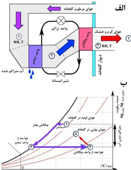
شکل ۴-۸: جریان هوا در یک پمپ حرارتی رطوبت‌زدا (الف) و تحول خواص هوای مرتبط به‌هنگام اجرای عملیات (ب) (شانتوی‌زو و همکاران، ۲۰۱۶)
