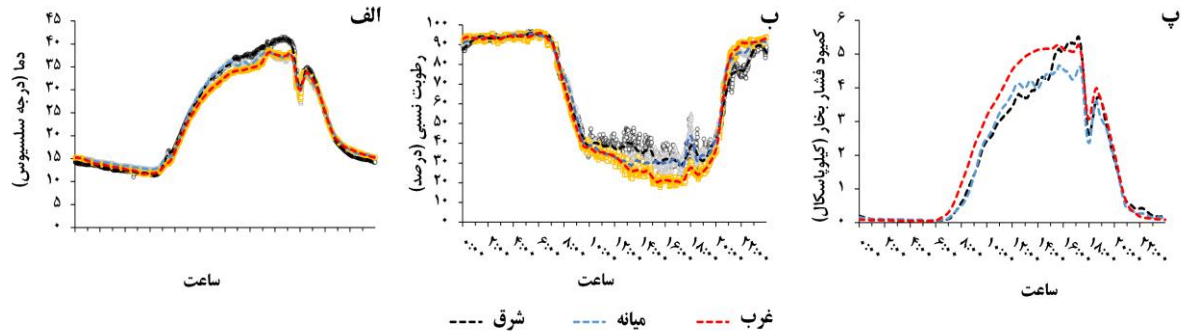
شکل ۳-۱۹: نمودار دما (الف)، رطوبت نسبی (ب)، کمبود فشار بخار (پ) در امتداد محور مرکزی عرضی یک گلخانه در تاریخ ۱۳۹۷/۰۳/۲۰ (رضوانی، ۱۳۹۹)
