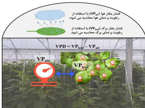
شکل ۱-۶: کمبود فشار بخار (آرگس، ۲۰۱۸؛ فاوست ۲ ، ۲۰۱۷؛ نگارندگان)
