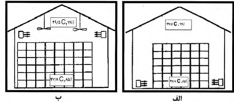
شکل ۱۳ - خشک کردن پس از برداشت خانواده پیازها با هوای گرم الف) منبع گرم کننده قسمت پایین محصول ب) منبع گرم کننده و دمنده قسمت بالای محصول
