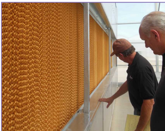
شکل ۴۰- نصب پد در دیواره طولی گلخانه
