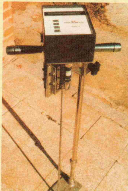
شکل ۲- دستگاه نفوذسنج مخروطی
