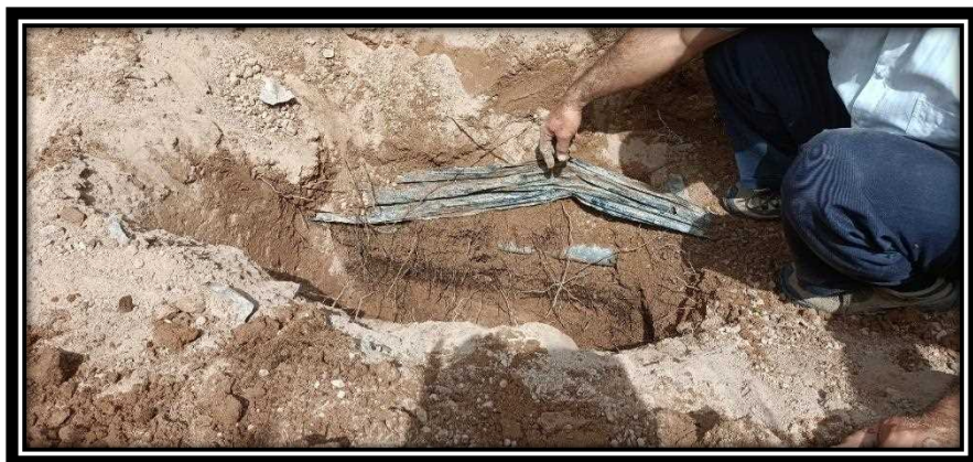
تصویر ۲۵- تجمع ریشه در اطراف لوله آبدۀ در منطقه انار (پایلوٹ ۱۰ ساله روی درختان مسن)
