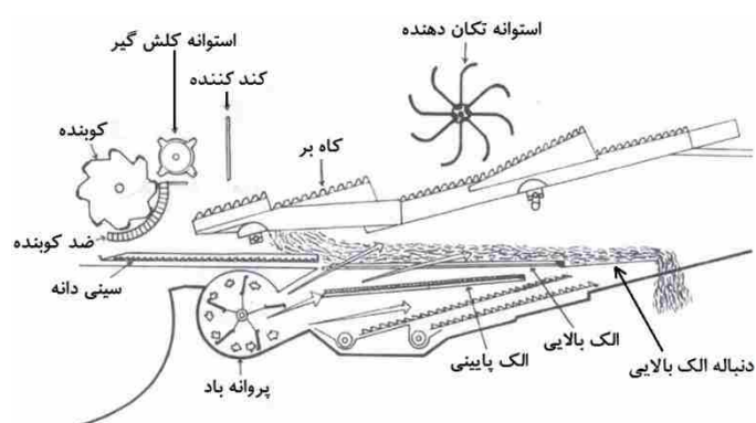
شکل ۹۷- استوانه تکان‌دهنده و کندکننده
