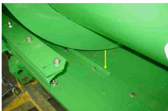
شکل ۱۰۹- فاصله هلیس تا کف سکو
