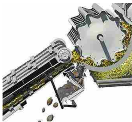
شکل ۹۱- سنگ‌گیر
