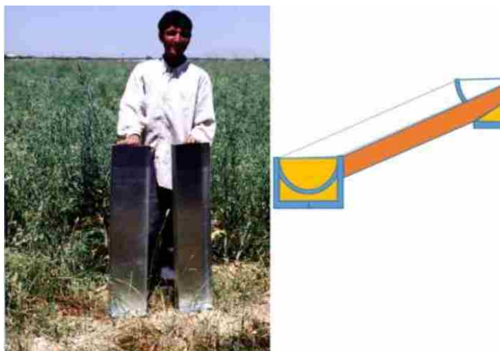
شکل ۱۱۵- ناودانی به ابعاد ۲۵×۱۰۰ سانتی متر برای اندازه‌گیری تلفات طبیعی محصول
