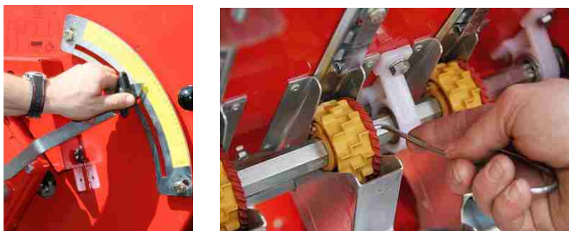
شکل ۵۹- تنظیم موزع‌های دستگاه برای بذرهای ریز
