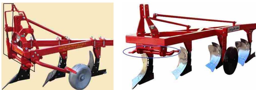
شکل ۲۶- تنظیم عرض کار در گاواهن‌های سه‌خیش سوارشونده
