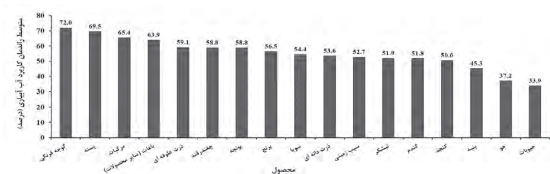
شکل ۷-۱- الف) فراوانی داده و ب) راندمان کاربرد آب آبیاری محصولات باغی و زراعی
